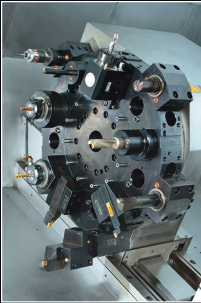
TORRETA BMT65 en TC800-110HL
